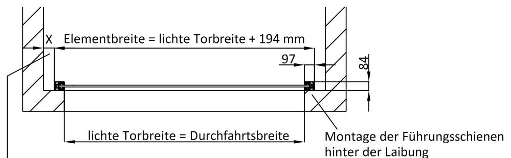
Schnittansicht
